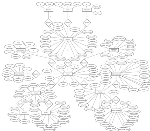
Gambar 6. ERD sistem
